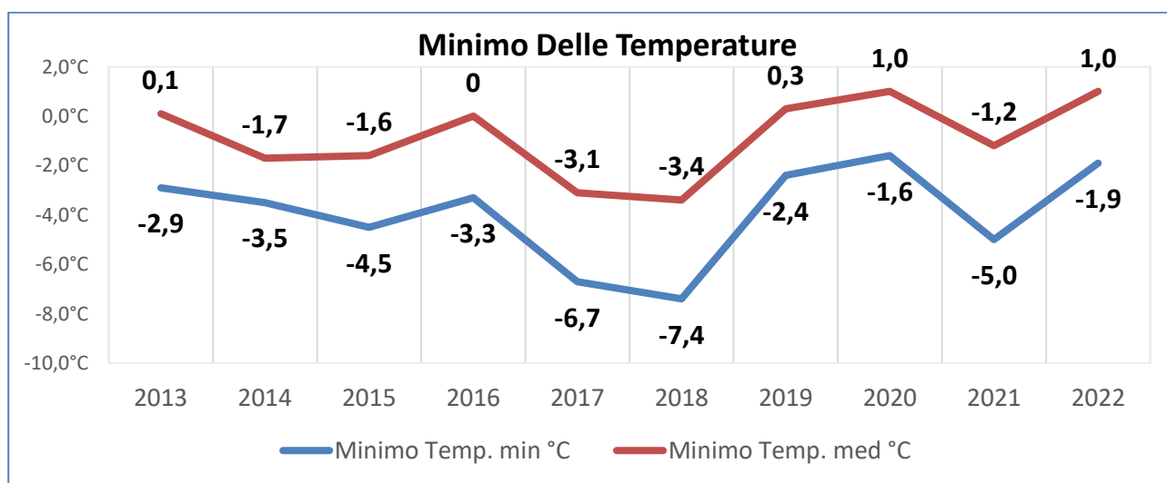
Grafico 7 - Minime Temperature annuali delle minime giornaliere e delle medie giornaliere nel periodo [2013-2022]
