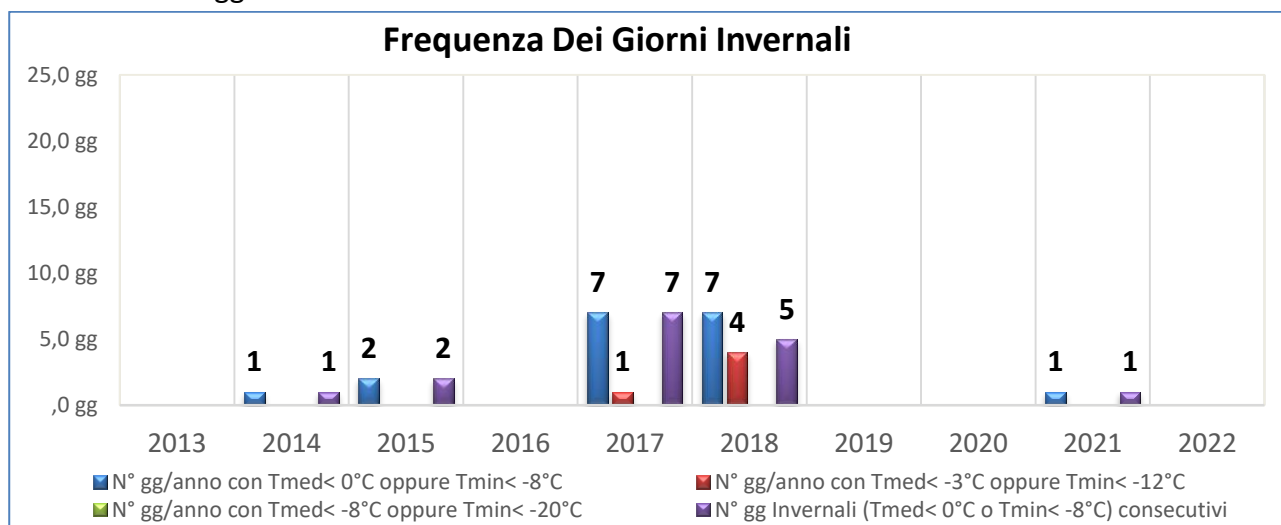
Grafico 8 – Massimo numero di giorni all'anno e Massimo numero di giorni consecutivi all'anno con Temperatura media/minima giornaliera inferiore ai limiti della classe di pericolosità Freddo Estremo nel periodo [2013-2022]
