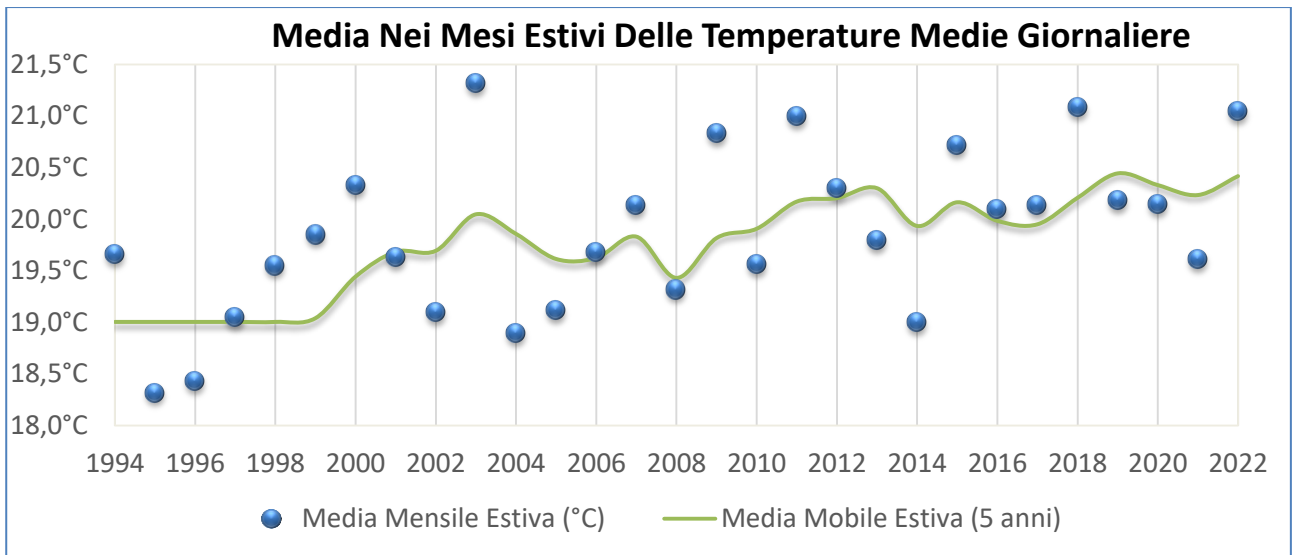
Grafico 4 - Media della Temperatura media giornaliera nei mesi estivi [1994 – 2022]
