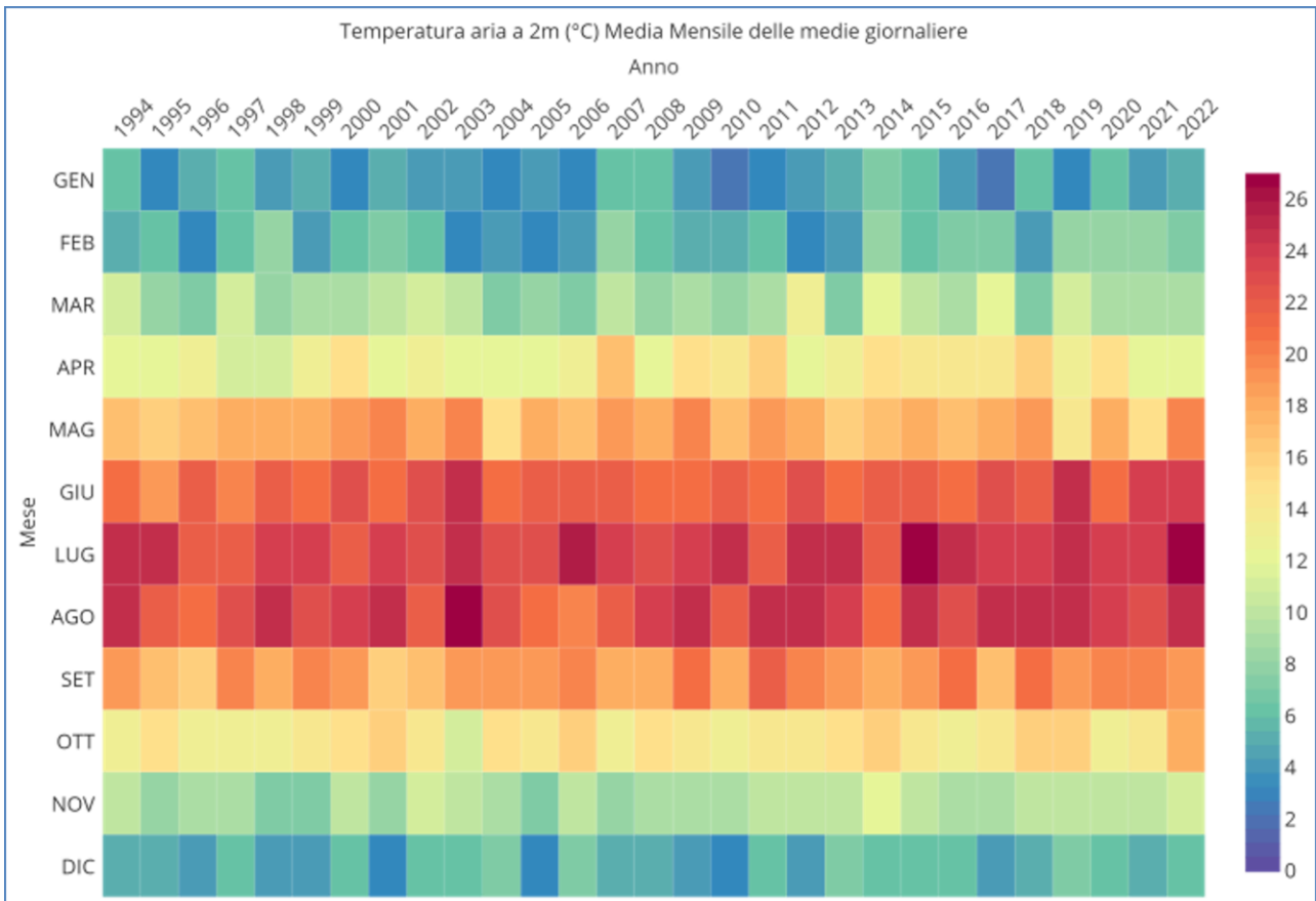
Grafico 9 - Media mensile della Temperatura media giornaliera [1994 – 2022]
