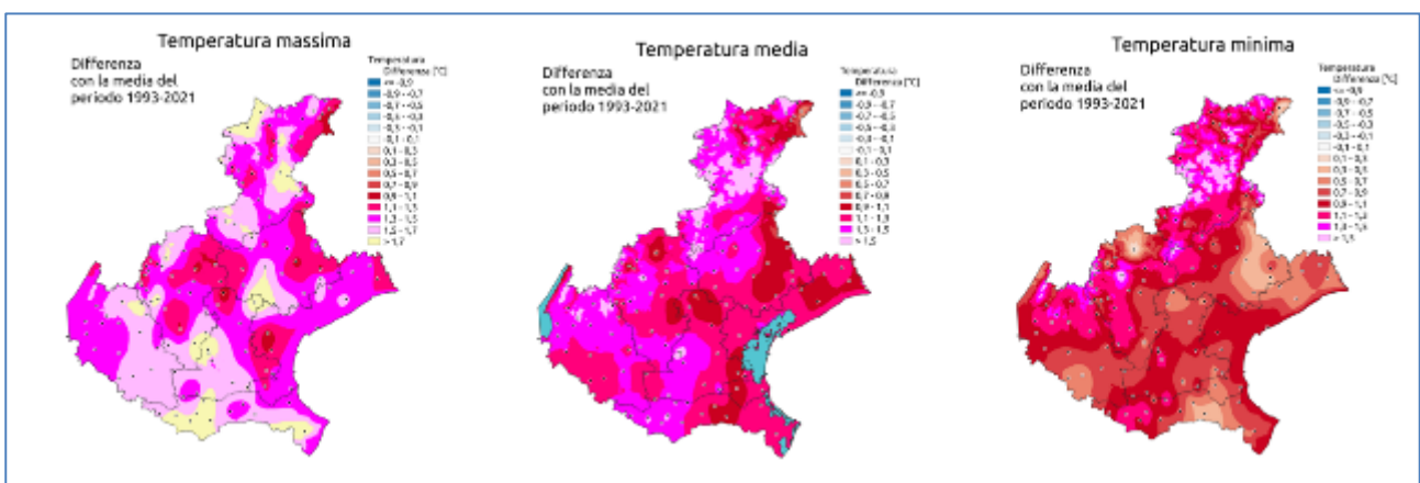
Figura 1 Andamento delle temperature nella regione Veneto - FONTE: ARPAV
