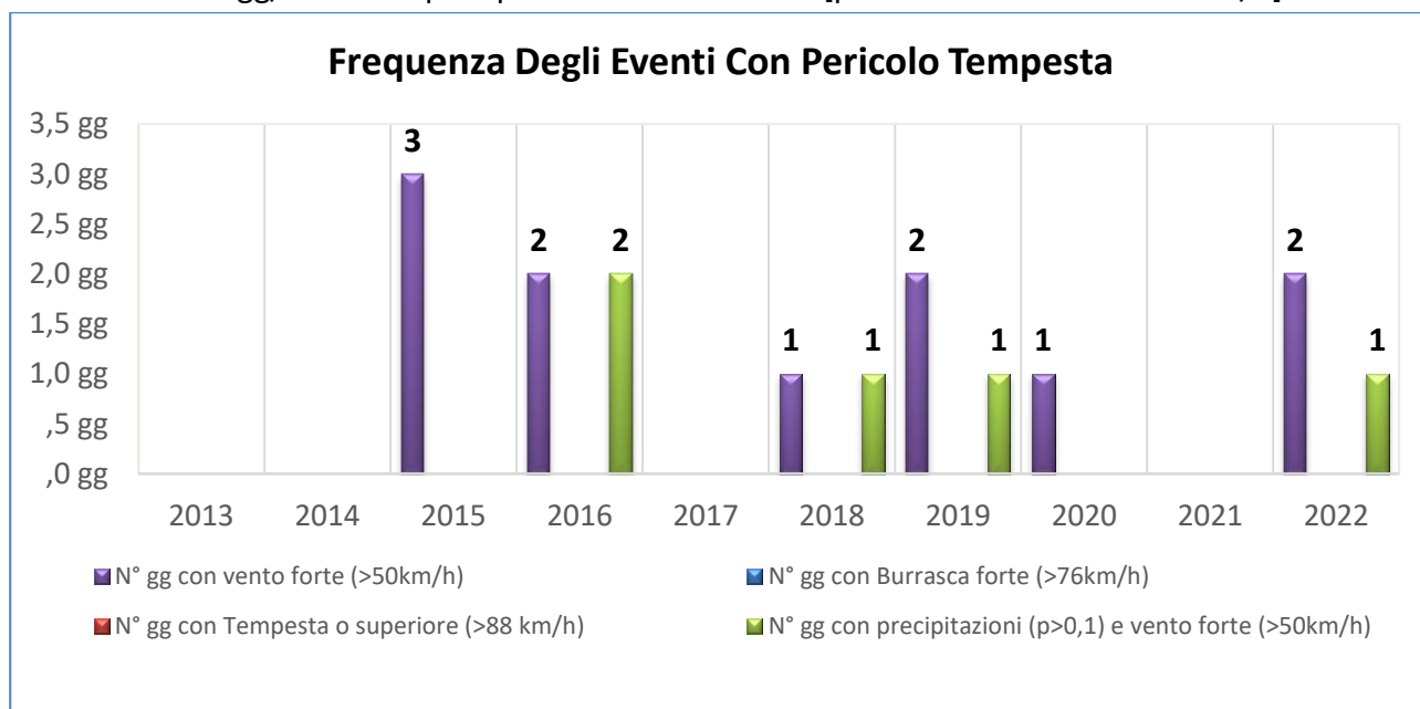
Grafico 22 – Frequenza degli eventi di pericolo Tempesta per grado di pericolosità [2013 – 2022]
