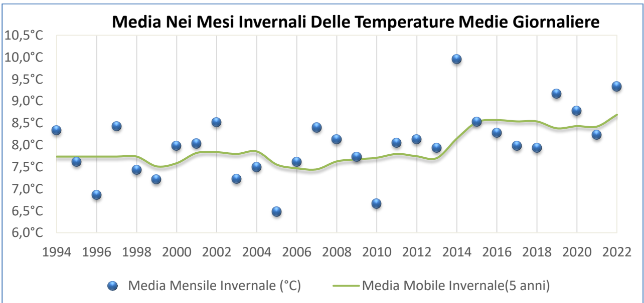
Grafico 10 - Media delle medie mensili delle Temperatura media giornaliera nei mesi invernali [1994 – 2022]
