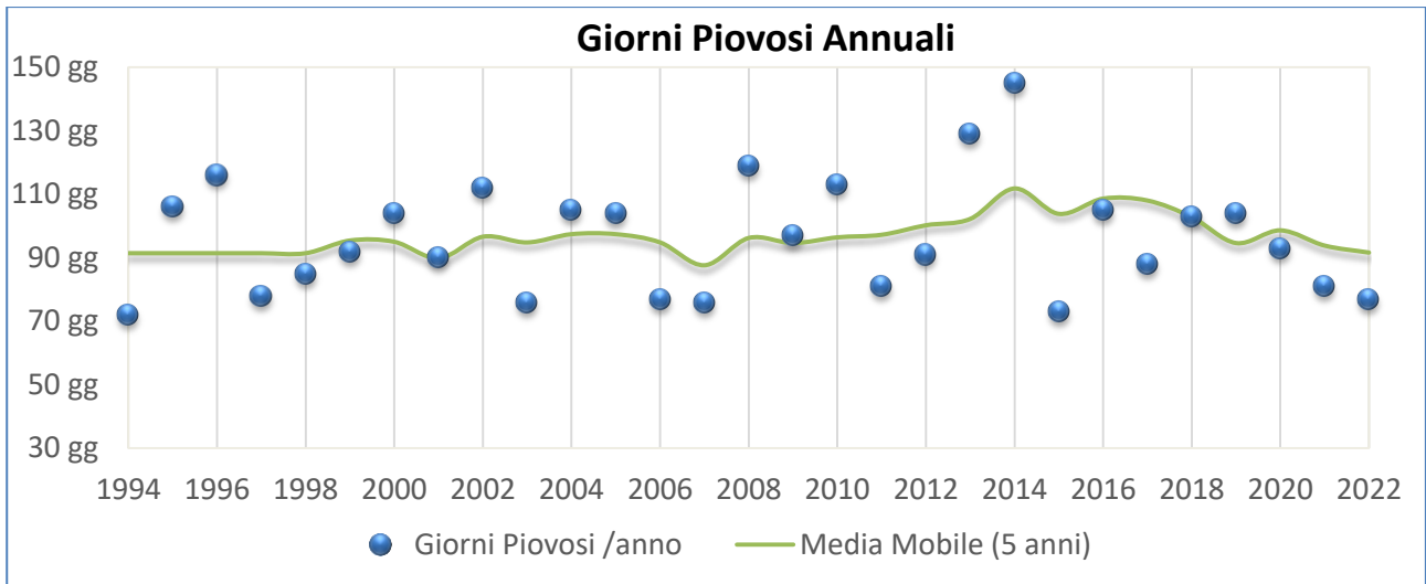
Grafico 16 – Numero di giorni piovosi all'anno nel periodo [1994-2022]
