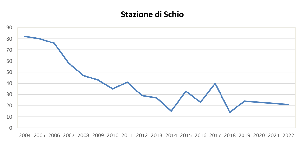
Grafico 23 – Giorni di superamento dei limiti di concentrazione di PM10 in atmosfera per le stazioni di rilevamento della provincia di Vicenza (gg/anno) [2004 - 2022]
