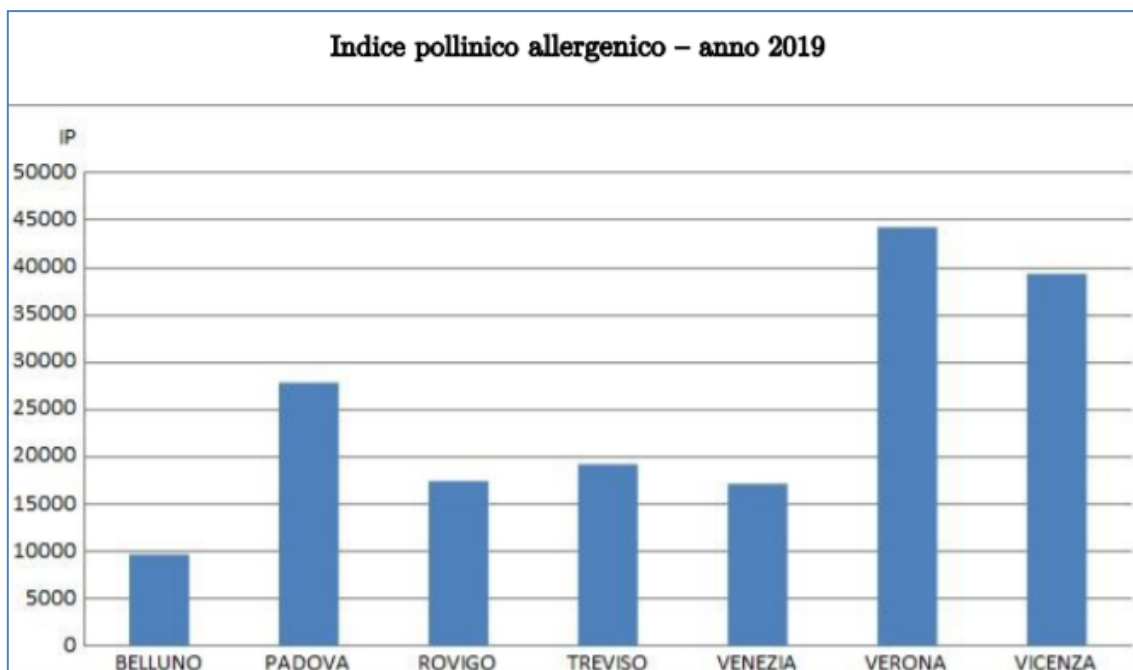
Figura 11 - Indice pollinico allergenico 2019 (Rapporto sullo Stato dell'ambiente del Veneto -Anno 2020)
