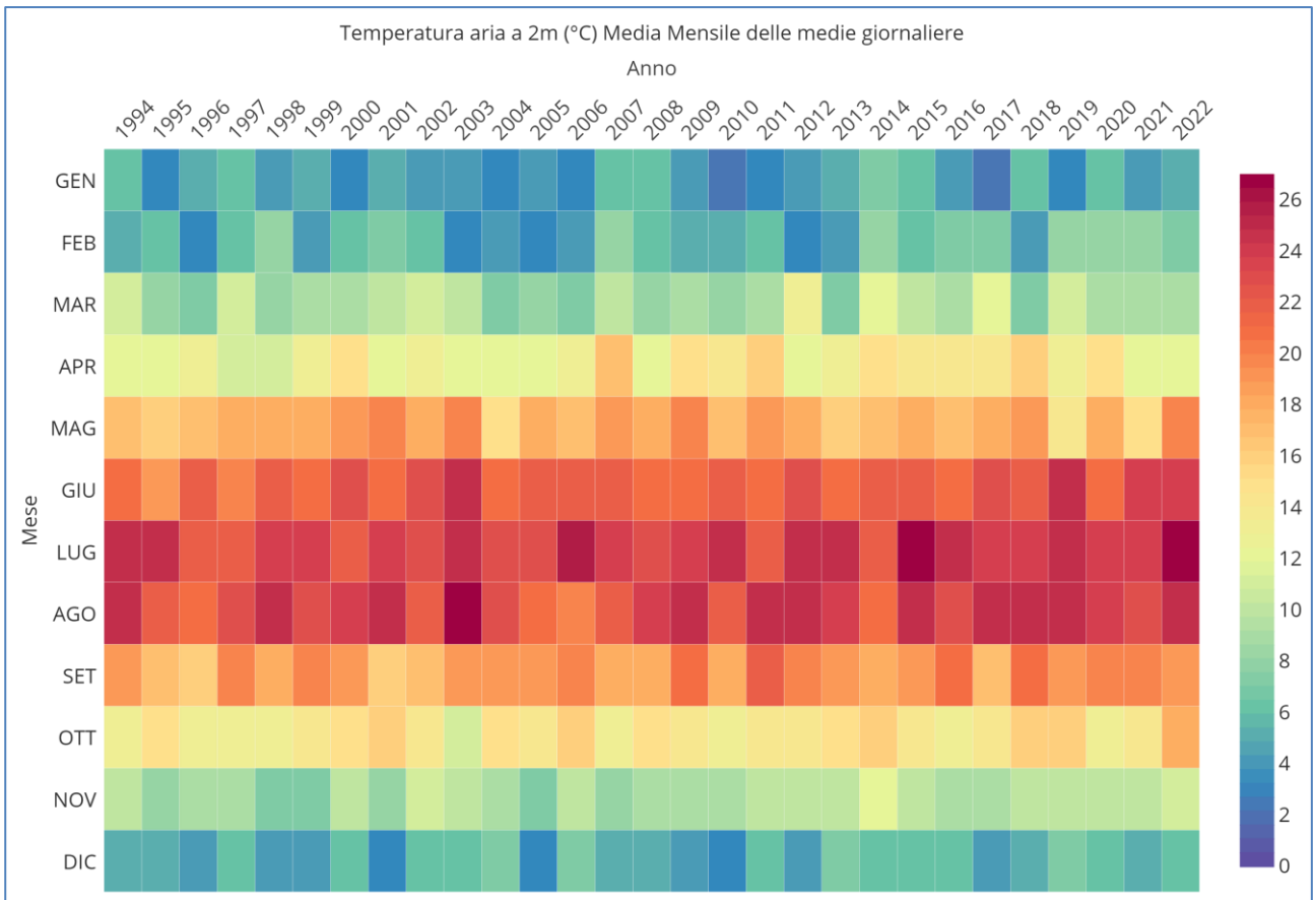
Grafico 3 - Media mensile della Temperatura media giornaliera [1994 – 2022]
